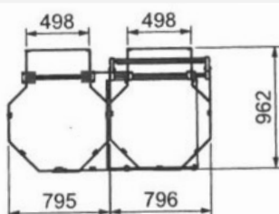
Arceau de protection avec changement de volée
